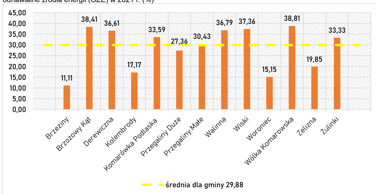
Wykres 82 Wskaźnik delimitacyjny nr 6 -sfera techniczna - Udział budynków mieszkalnych wykorzystujących odnawialne źródła energii (OZE) w 2021 r. (%)
