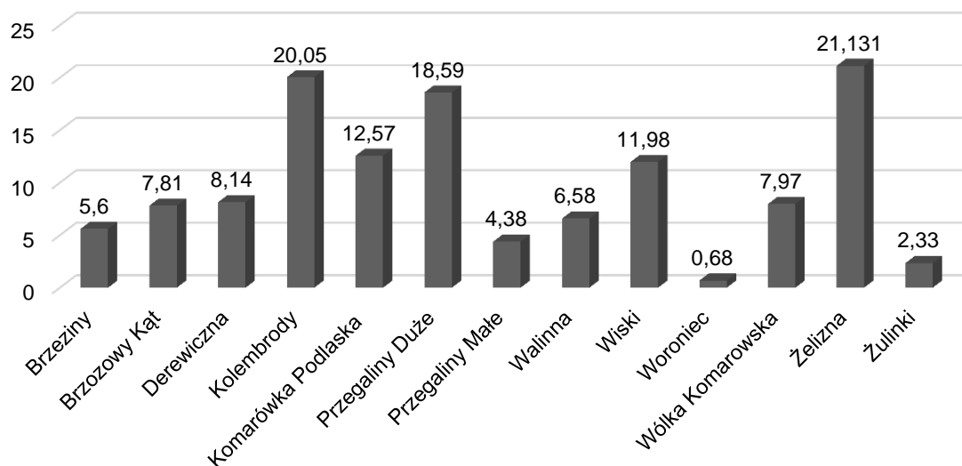
Wykres 88 Długość dróg lokalnych na terenie gminy Komarówka Podlaska w 2021 r. wg jednostek referencyjnych (km)
