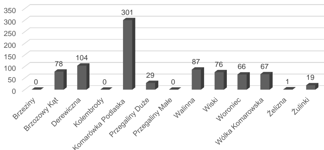
Wykres 80 Charakterystyka wyposażenia budynków mieszkalnych w infrastrukturę wodociągową na terenie gminy Komarówka Podlaska w 2021 r. wg podziału na jednostki referencyjne
