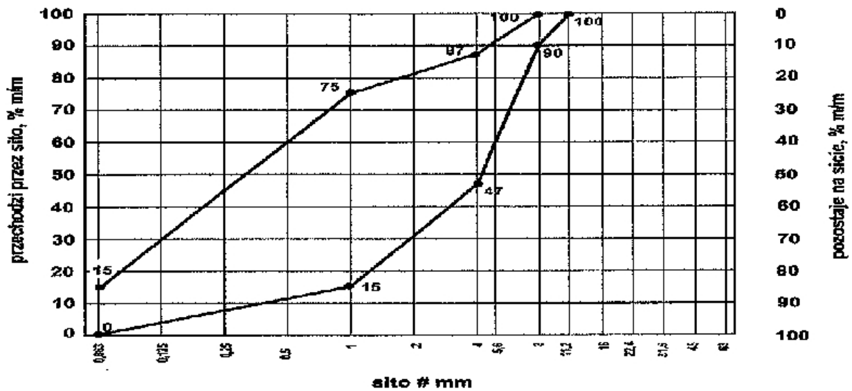
Rysunek 2 Mieszanka niezwiązana 0/16 do dolnej warstwy nawierzchni ścieżki rowerowej, dróg leśnych oraz poboczny
