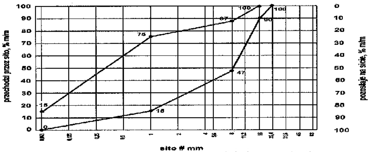
Rysunek 2 Mieszanka niezwiązana 0/16 do dolnej warstwy nawierzchni ścieżki rowerowej, dróg leśnych oraz poboczny
